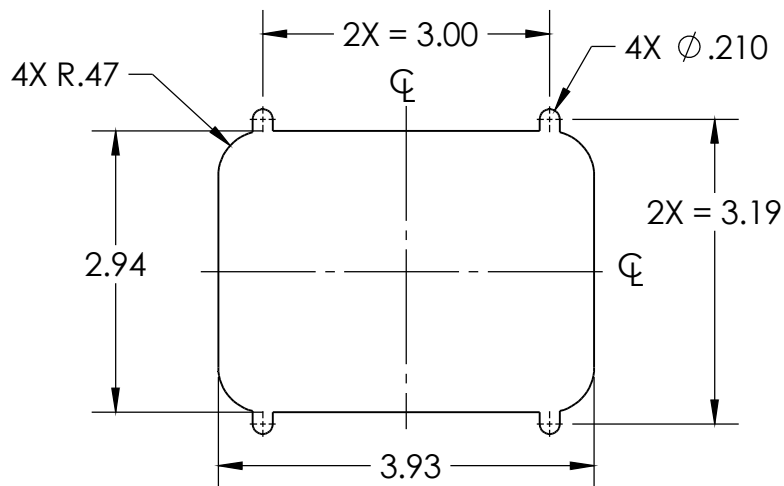
T-HANDLE CUTOUT
