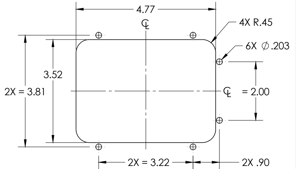
T-HANDLE CUTOUT
