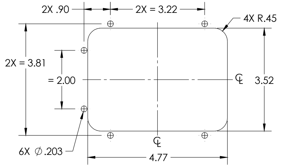
T-HANDLE CUTOUT
