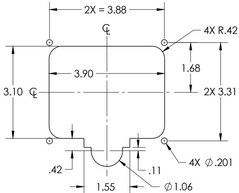
T-HANDLE CUTOUT
